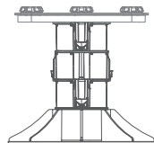
P 9236 + 3x P 9241 + P 9243 (= MAX) min. 185 mm – max. 225 mm
