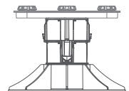
P 9236 + 2x P 9241 + P 9243 min. 145 mm – max. 185 mm
