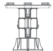
P 9236 + 3x P 9241 + P 9247 (= MAX) min. 185 mm – max. 225 mm
